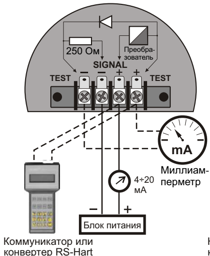
Исполнения: APC-2000AL APC-2000ALW
