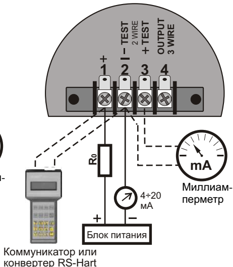
Исполнение APC-2000ALE с выходом 4...20 мА
