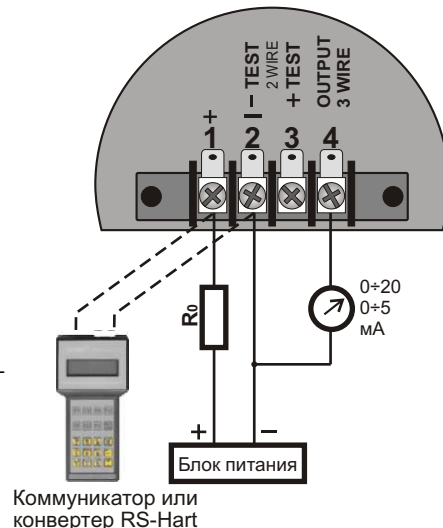
Исполнение APC-2000ALE с выходом 0...5 или 0...20 мА
